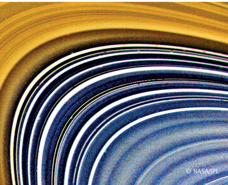
Saturn, Detailaufnahme des C-Rings
